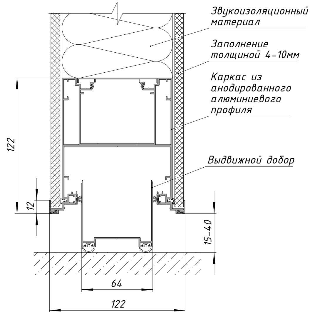
Узел примыкания к полу
