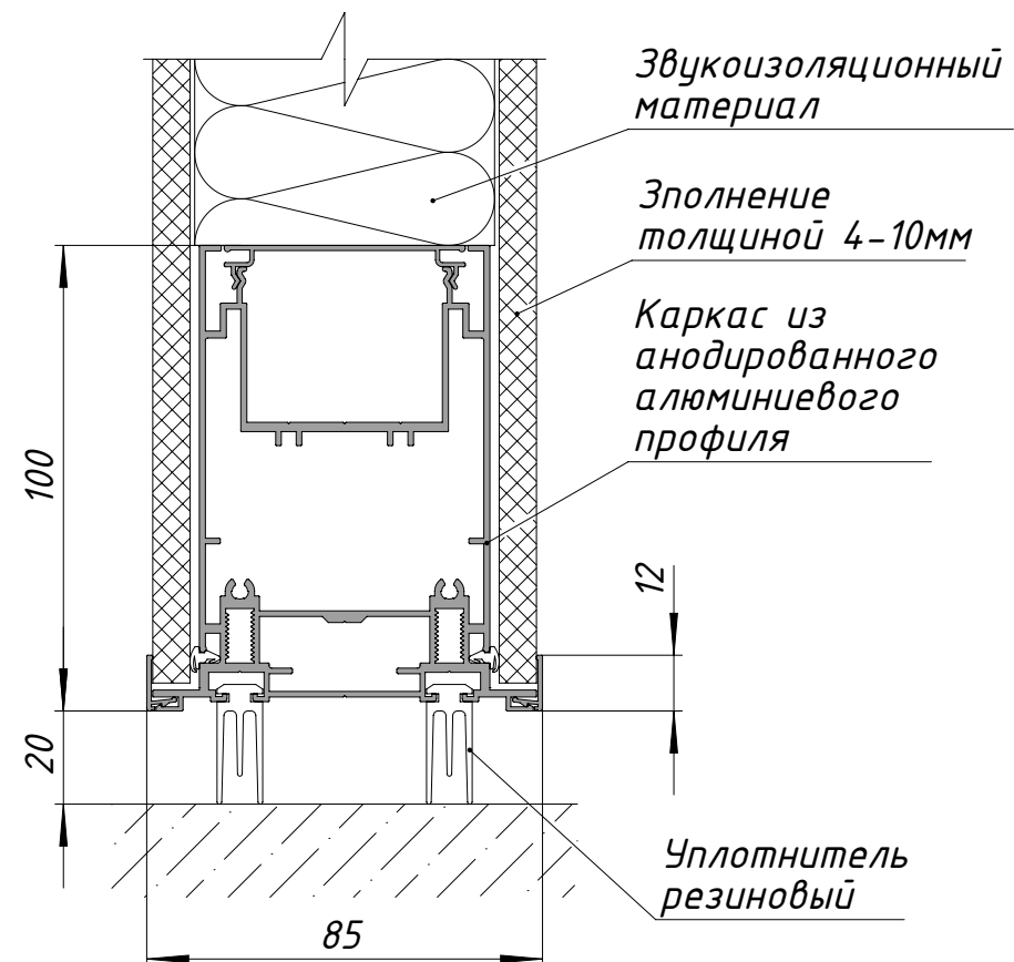
Узел примыкания к полу
